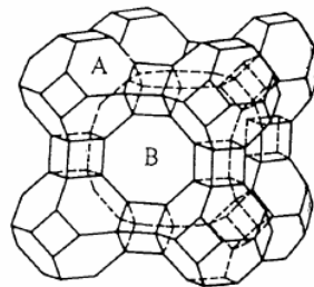
Gambar 4.10 Struktur zeolit A.
