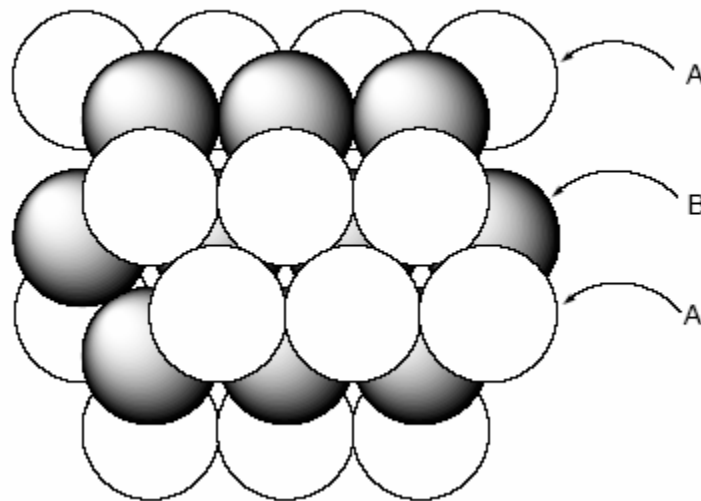
Gambar 2.2 Susunan hcp bola.
