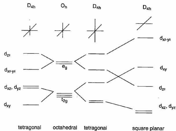
Gambar 6.7 Perubahan energi orbital dari koordinasi oktahedral ke bujur sangkar.
