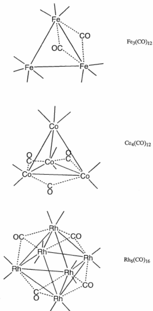
Gambar 6.23 Contoh karbonil kluster logam (ligan karbonil terminal dihilangkan agar terlihat jelas).
